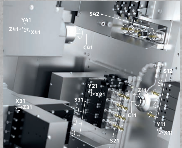
EvoDECO 20 & EvoDECO 32
